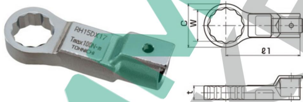
RH15Dx17 - общий вид
